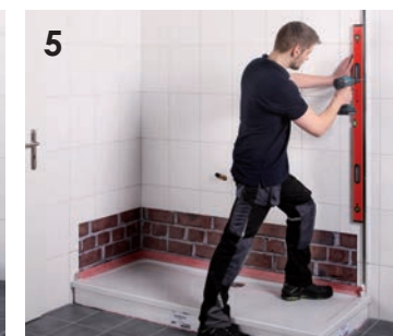
5 Installation der Vorwandmontage.
