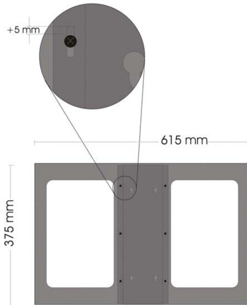
Befestigungsrahmen
