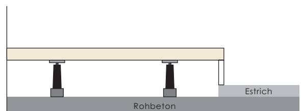
Montage auf Montagerahmen
