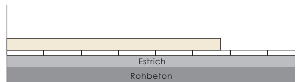
Montage auf fertig gefliesten Boden
