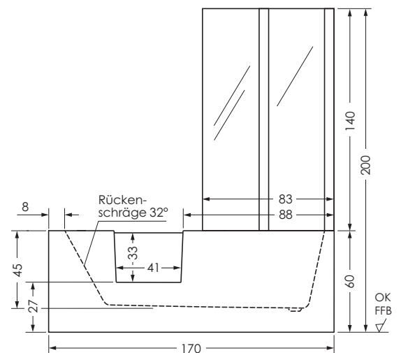
Seitenansicht
