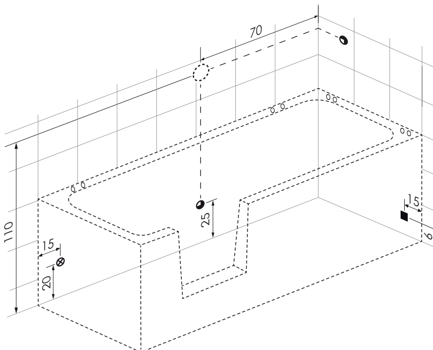
Standfläche / Wasseranschlüsse
