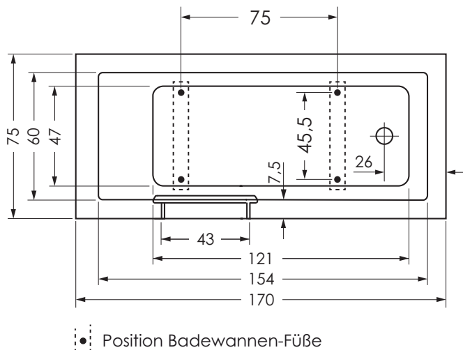
Draufsicht
