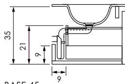
BASE 45 + Waschtischplatte
