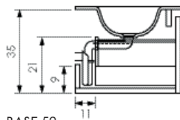
BASE 52 + Waschtischplatte
