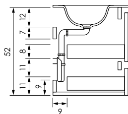
BASE 45 WP + Waschtischplatte
