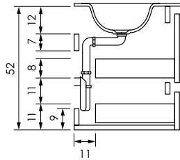
BASE 52 WP + Waschtischplatte
