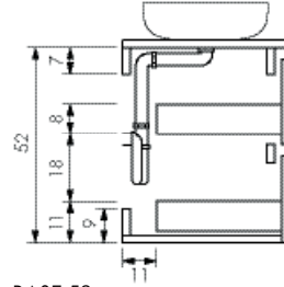
BASE 52 + Abdeckplatte / Aufsatzwaschtisch
