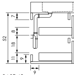
BASE 45 + GENF
