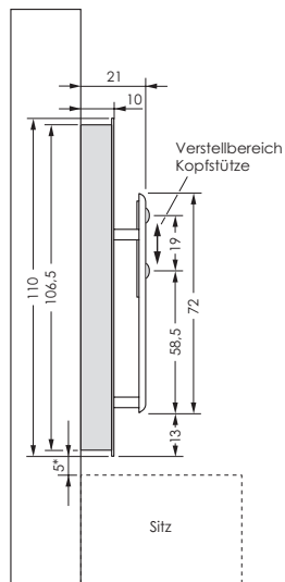
Seitenansicht
