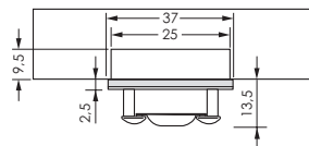
Draufsicht
